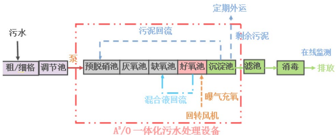
图 2.1-1 A 3 /O-MBBR 一体化工艺污水处理工艺流程图
